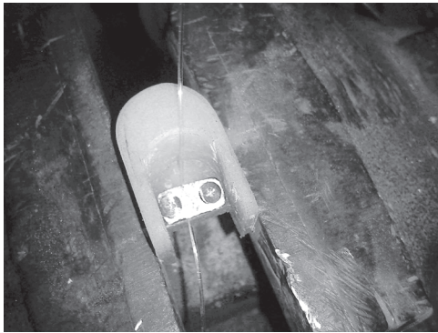
Fig. 19. Ajuste de hilo nailon Fuente: Autoría propia
