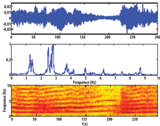
Figura 2. Otro tipo de tremor en que se observan claramente la presencia de armónicos, así como la brusca caída de éstos a la mitad de su valor en frecuencia, fenómeno conocido como desdoblamiento espectral.
