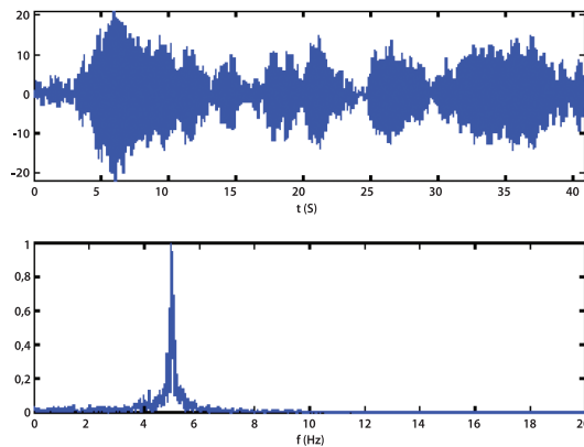
Figura 6. Solución numérica por el método de Runge-Kutta de la ecuación que describe el proceso de turbulencia elástica. Para el ejemplo se eligió una frecuencia fundamental de 5 Hz que se recupera bien en el espectro de Fourier. Podemos ver que la forma y el espectro de la señal obtenida se corresponden con la esperada para un tremor volcánico mono-frecuencial.
