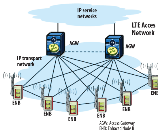
Figura 2. Arquitectura de red de acceso LTE.
