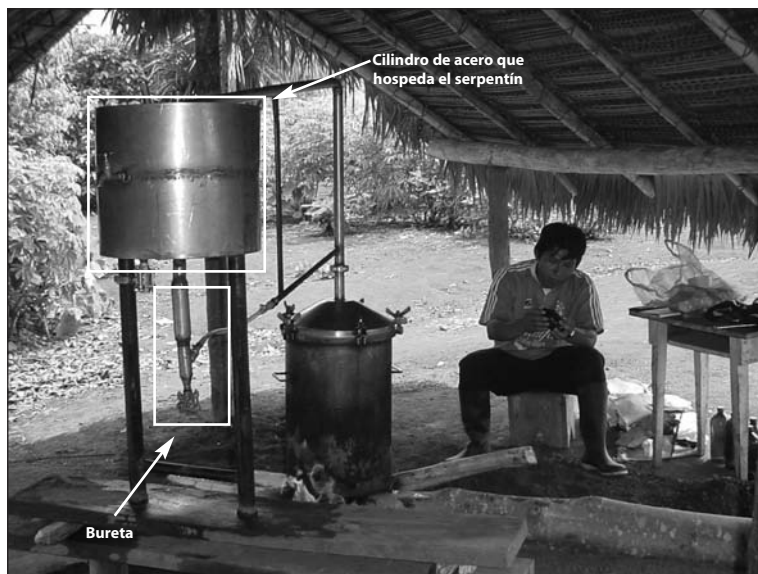
Destilador con sistema discontinuo de enfriamiento comunidad Trans-Kutuku
