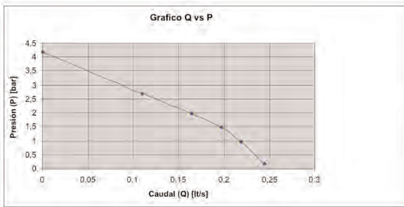
Figura 15. Curva característica motriz H-Q de la bomba de ariete hidráulico con una válvula de impulso
