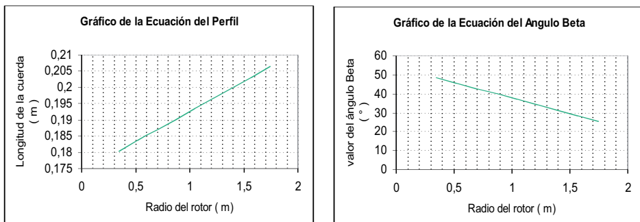
Fig. 11 a) Gráfico de la Ecuación del Perfil del álabo, mostrando la longitud de la cuerda en función del radio del rotor, b) Se muestra la variación del ángulo beta en función del radio del rotor.
