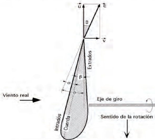
Figura 10. Gráfica del álabo con las condiciones calculadas.
