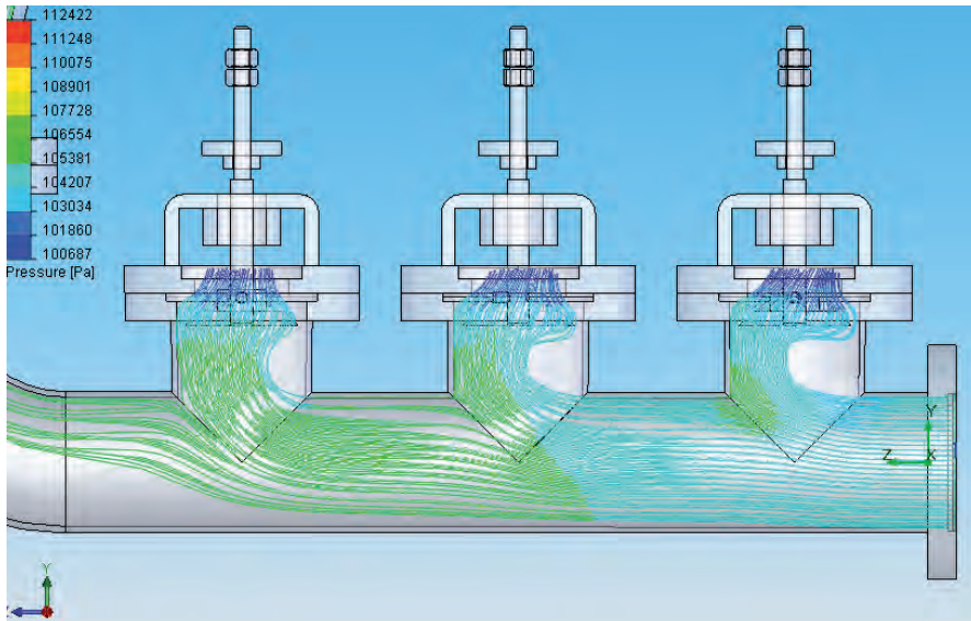
Figura 8. Diagrama de presiones dinámicas de válvulas de impulso de Ariete Hidráulico
