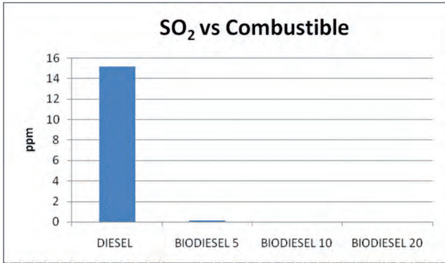
Fig.5 Comportamiento del SO 2 en función de la adición del biodiesel.
