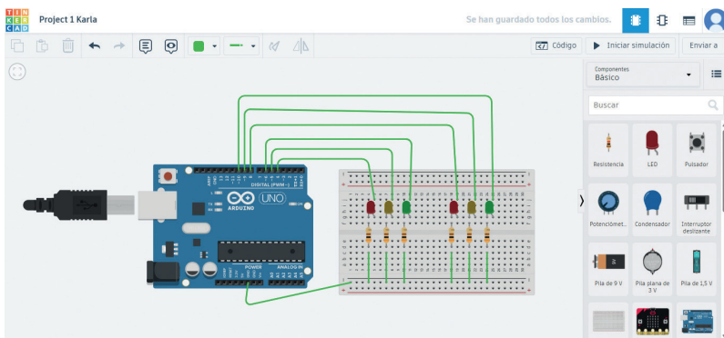
FIGURA 21 Prototipo de circuito digital en Tinkercad
