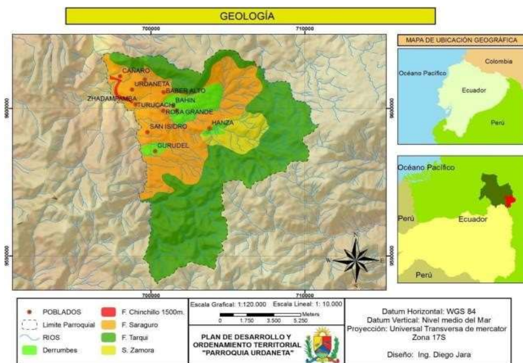
Figura 2. Mapa geológico.
