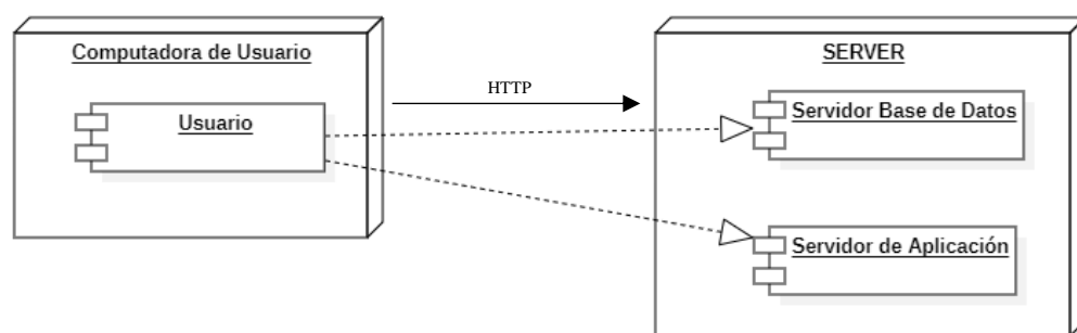
Figura 15. Esquema de despliegue para la infraestructura de la aplicación Web.
