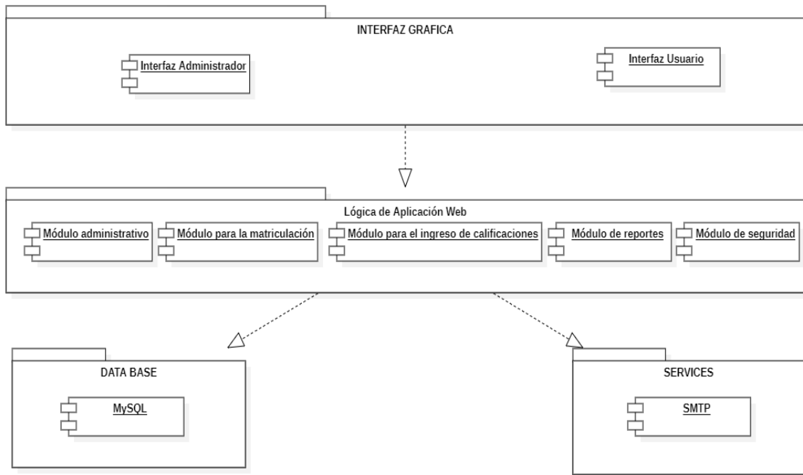
Figura 8. Esquema de componentes para la aplicación Web Fuente: Elaboración propia de los autores
