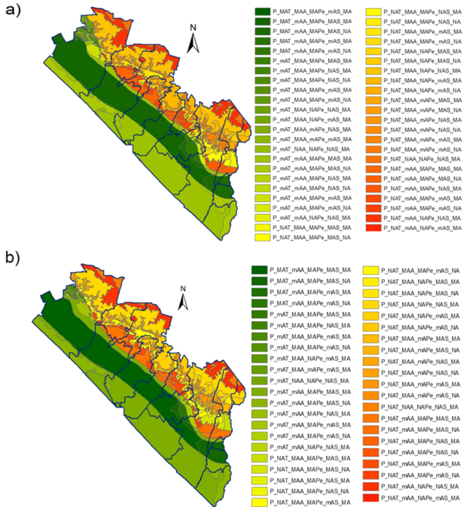
Figura 9. Aptitud futura por limitantes a) modelo GFDL A2 y B2, b) modelo Hadley A2 y B2 para cacao en escenarios de cambio climático en la región del Soconusco, Chiapas, México.
