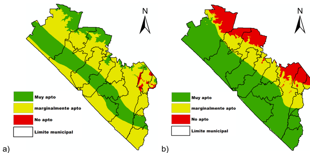
Figura 4. Aptitud actual de la tierra con el método de ponderación para café (a) y cacao (b) en la región del Soconusco, Chiapas, México.
