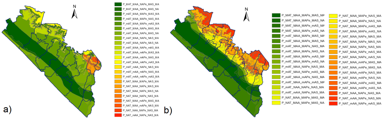
Figura 5. Aptitud actual de la tierra con el método de limitantes para café (a) y para cacao (b) en la región del Soconusco, Chiapas, México.
