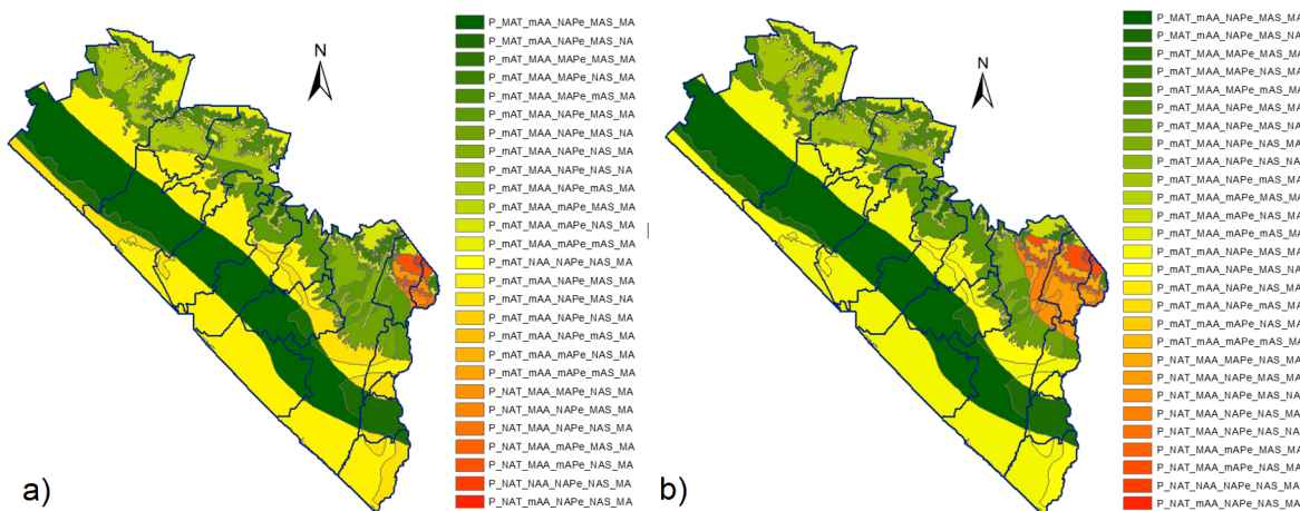
Figura 8. Aptitud futura por limitantes a) modelo GFDL A2 y B2, b) modelo Hadley A2 y B2 para café en escenarios de cambio climático en la región del Soconusco, Chiapas, México.
