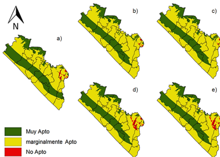
Figura 6. Zonificación para el cultivo de café: a) Aptitud actual y; Aptitud con escenarios de cambio climático para el año 2030: b) GFDL A2, c) GFDL B2, d) Hadley A2 y e) Hadley B2.
