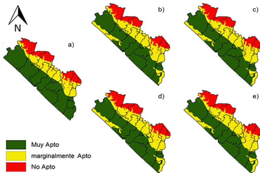
Figura 7. Zonificación para el cultivo de cacao: a) Aptitud actual y; Aptitud con escenarios de cambio climático para el año 2030: b) GFDL A2, c) GFDL B2, d) Hadley A2 y e) Hadley B2.
