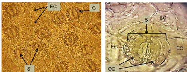
Figura 4. Detalles micromorfológicos de la hoja de Chuquiragua
