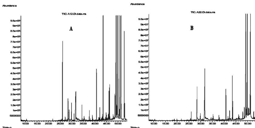
Figura 5. Perfiles cromatográficos de los extractos hexánicos de a) flores y b) hojas de Chuquiragua
