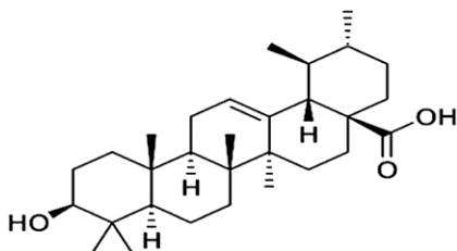
Figura 5. Estructura del compuesto ácido ursólico
