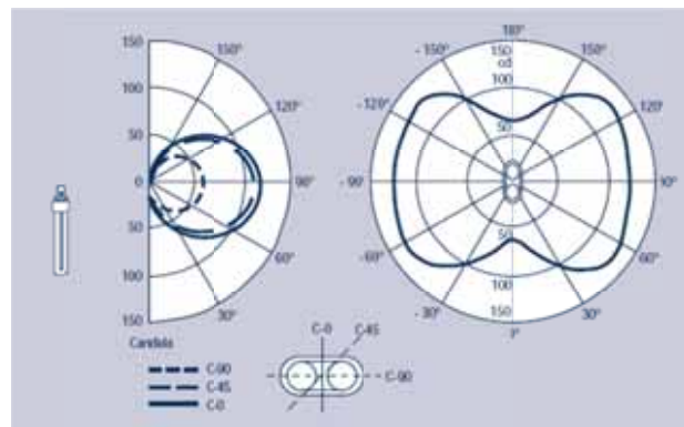
Figura 9. Lámpara OSRAM DULUX® S, OSRAM DULUX® S/E, OSRAM DULUX® L (Distribución de intensidad luminosa axial y radial referida a 1000)
