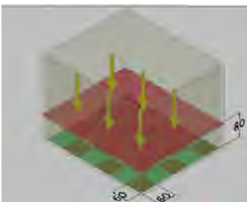
Figura 25. (Método para realizar la medición de los niveles de iluminación en una habitación)
