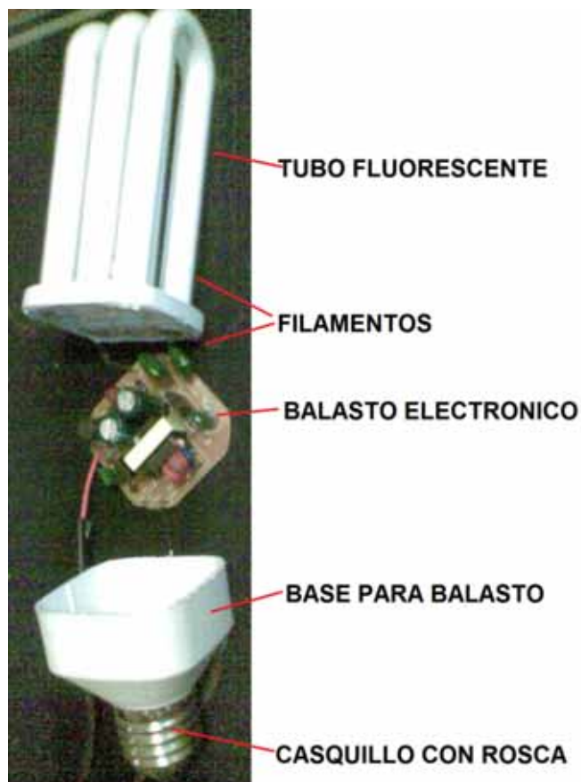
Figura 1. Partes del foco ahorrador
