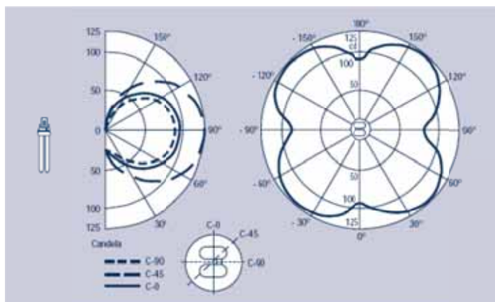
Figura 12. Lámpara OSRAM DULUX® D, OSRAM DULUX® D/E (Distribución de intensidad luminosa axial y radial referida a 1000)
