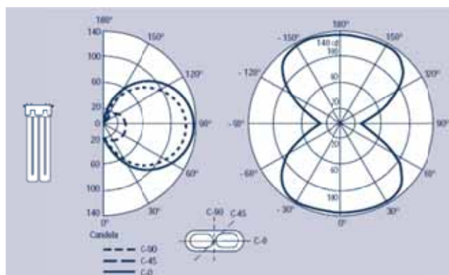
Figura 10. Lámpara OSRAM DULUX® F (Distribución de intensidad luminosa axial y radial referida a 1000)
