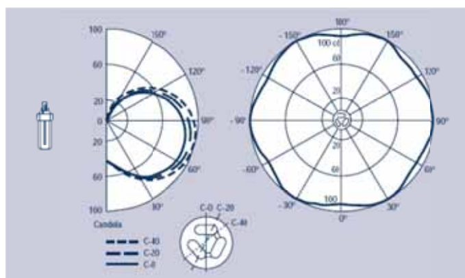
Figura 11. Lámpara OSRAM DULUX® T, OSRAM DULUX® T/E (Distribución de intensidad luminosa axial y radial referida a 1000)
