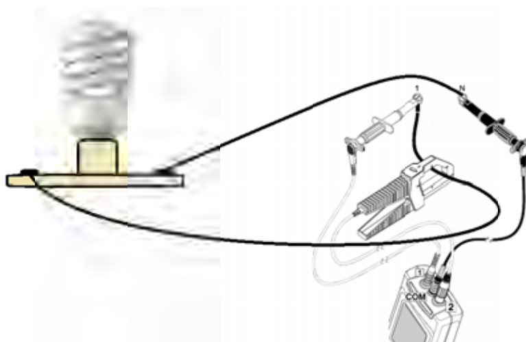
Figura 22. Medición de Potencia, factor de potencia.
