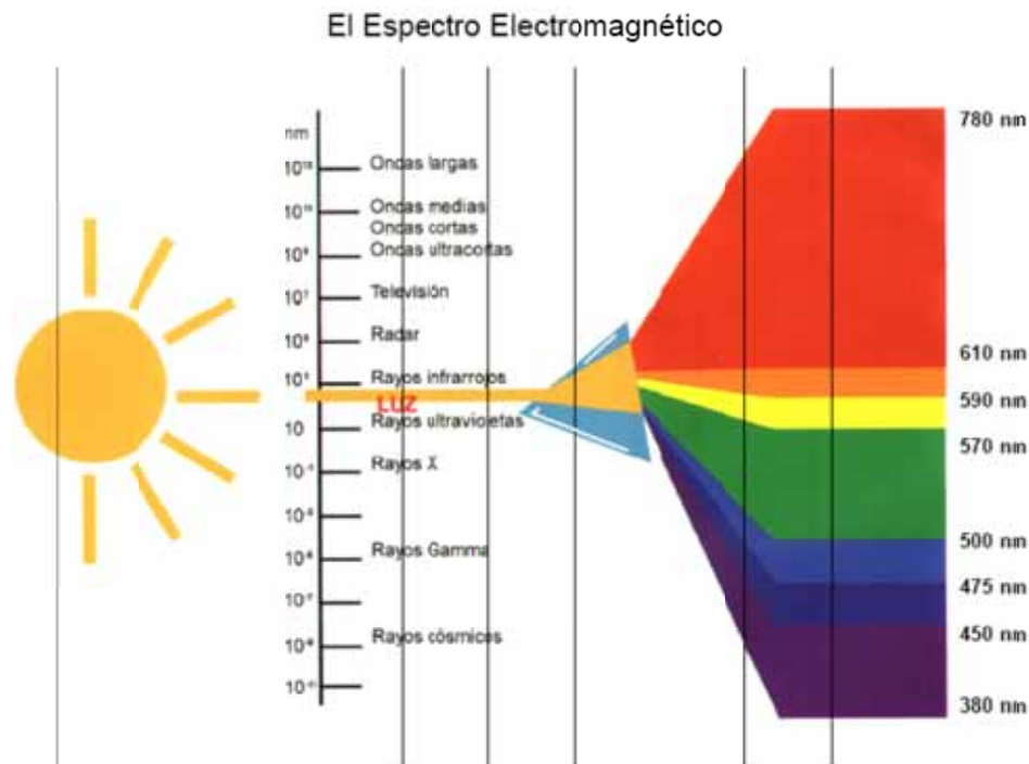
Figura 6. Espectro electromagnético 15
