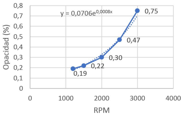
Figura 2. Porcentaje de opacidad B15
