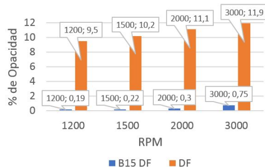
Figura 3. Gráficas comparativas diésel fósil y biodiésel B15
