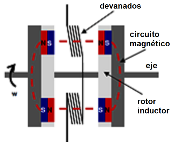
Figura 1. Vista transversal de un generador axial.
