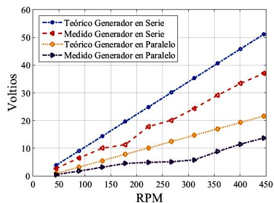
Figura 19. Comparaciones de voltajes teórico y medido.
