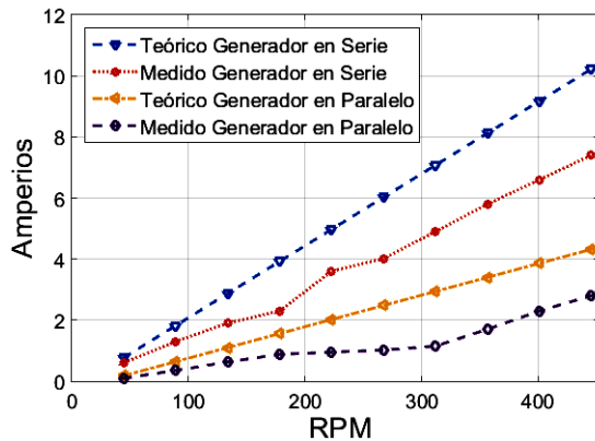
Figura 20. Comparaciones de amperajes teórico y medido.
