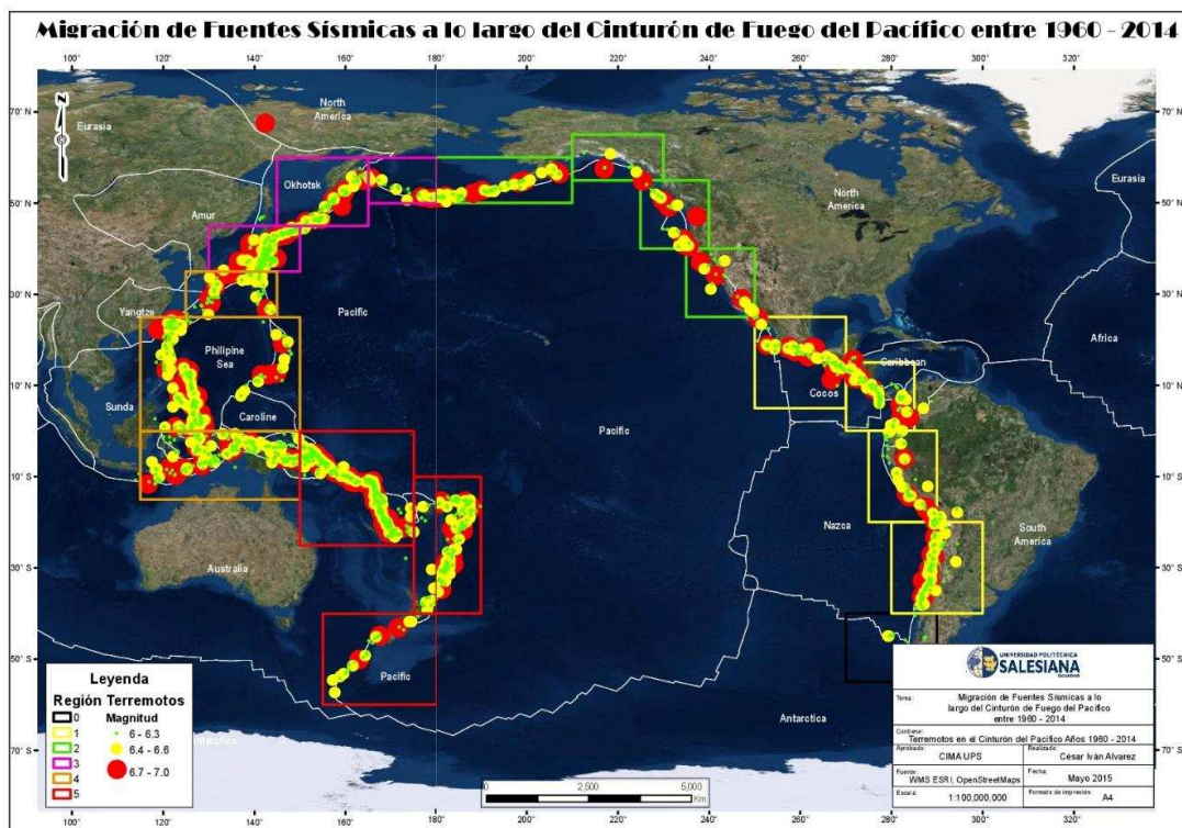
Figura 1. Distribución de epicentros sísmicos 1960-2014. Región 1: cuadros de color amarillo; Región 2: cuadros de color verde; Región 3: cuadros de color magenta; Región 4: cuadros de color naranja; Región 5: cuadros de color rojo.
