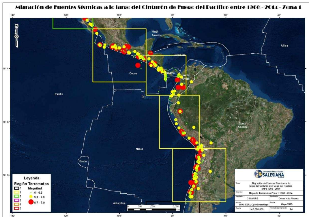
Figura 2. Distribución de epicentros sísmicos 1960-2014.
