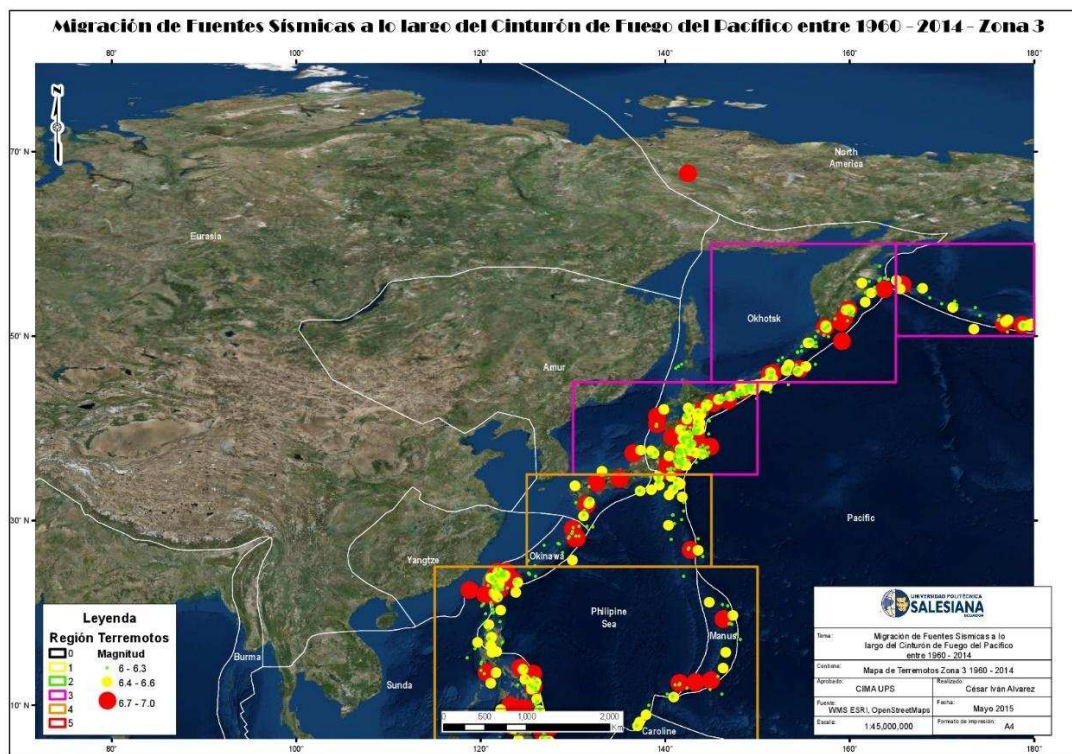
Figura 6. Distribución de epicentros sísmicos 1960-2014.
