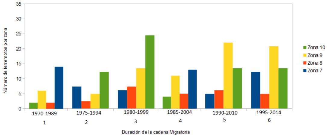
Figura 3. Distribución de terremotos en la Región 1.
