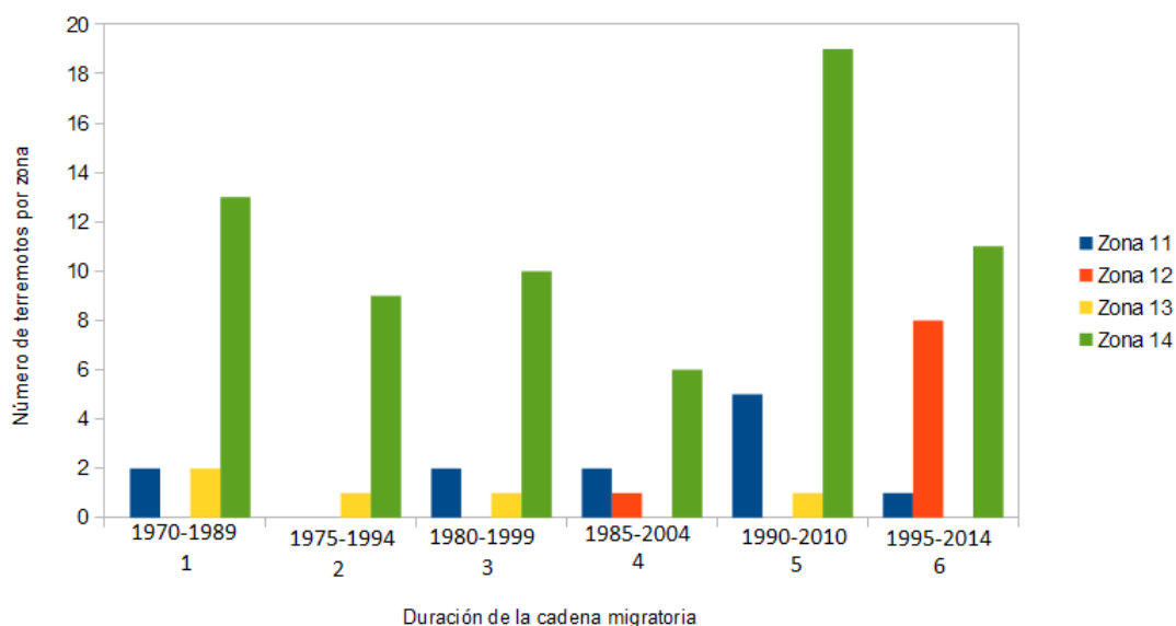
Figura 5. Distribución de terremotos en la Región 2.
