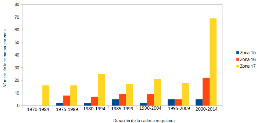
Figura 7. Distribución de terremotos en la Región 3.
