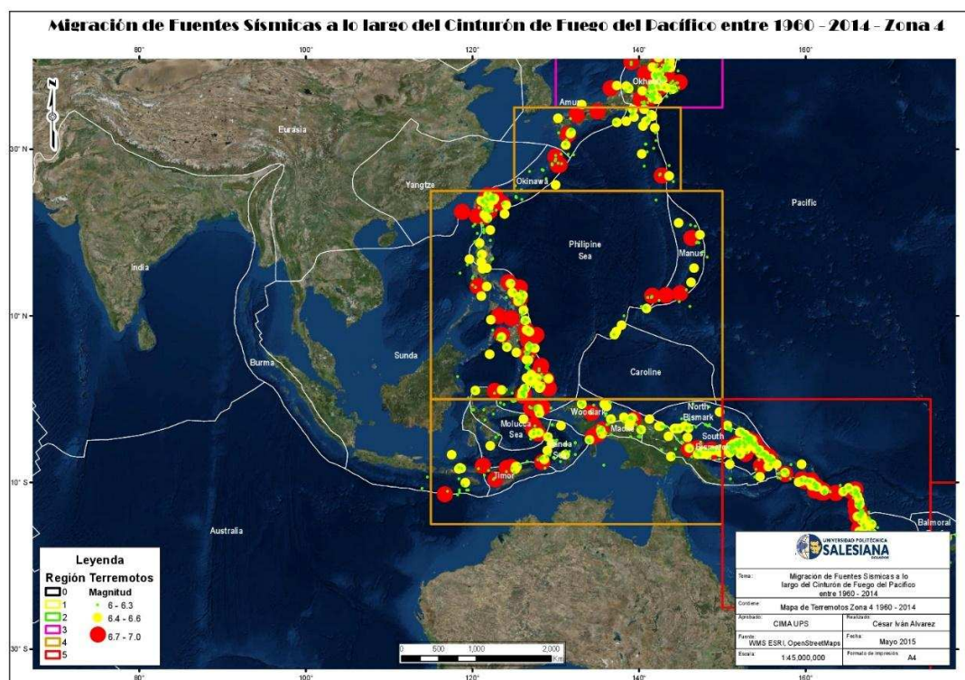
Figura 8. Distribución de epicentros sísmicos 1960-2014.
