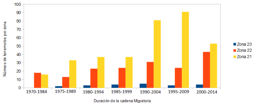
Figura 11. Distribución de terremotos en la región 5.
