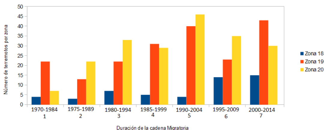
Figura 9. Distribución de terremotos en la Región 4.
