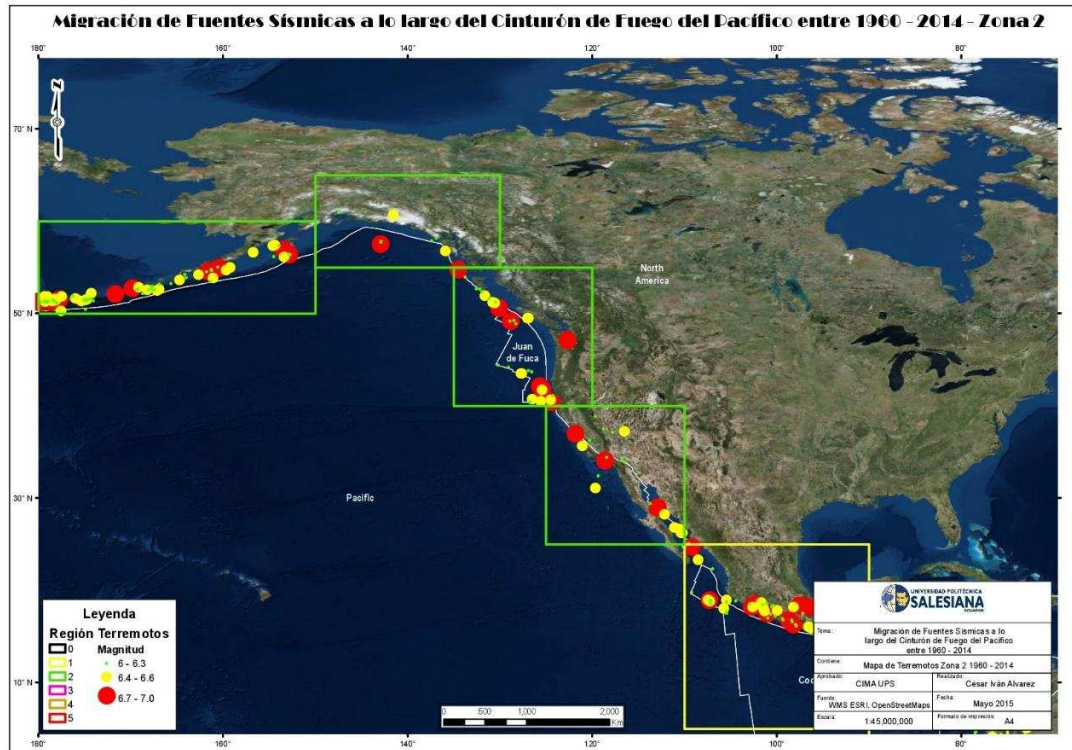
Figura 4. Distribución de epicentros sísmicos 1960-2014.
