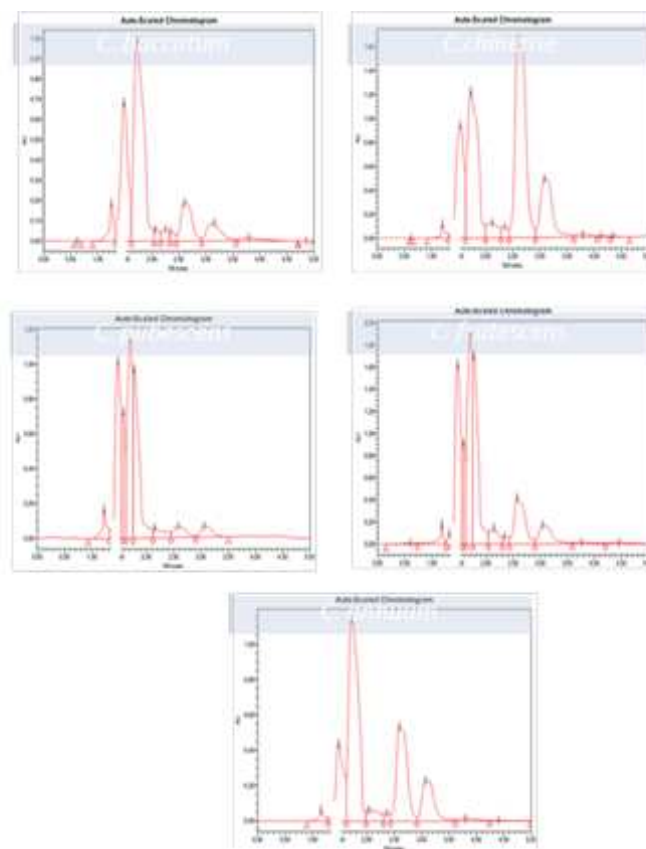
Figura 5. Cromatogramas de las muestras de las cinco especies de Capsicum .
