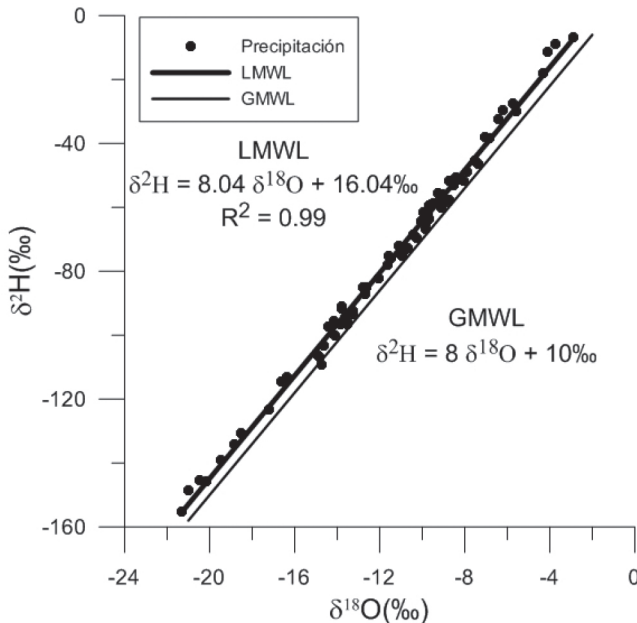
Figura 2 Relación entre los valores de \delta^{18}\text{O} y \delta^2\text{H} de las muestras de precipitación obtenidas en la cuenca del río Zhurucay
