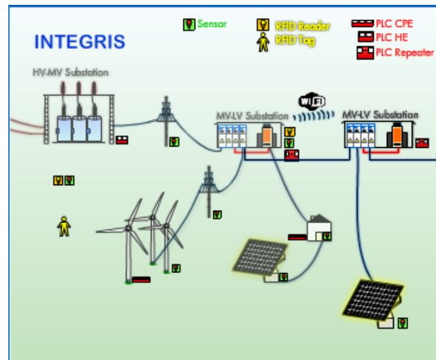
Figura 3. Proyecto planteado por Integris. [19]
