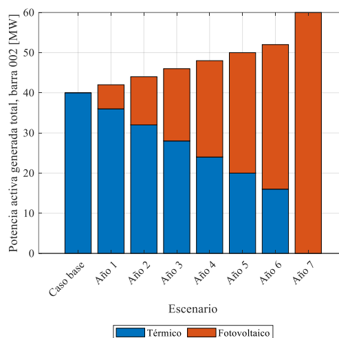
Figura 9. Generación combinada en la barra 2, cambio abrupto.
