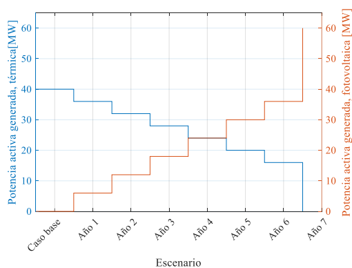
Figura 8. Disminución abrupta de generación térmica.
