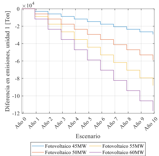
Figura 7. Diferencia de emisiones de CO 2 , unidad 1.
