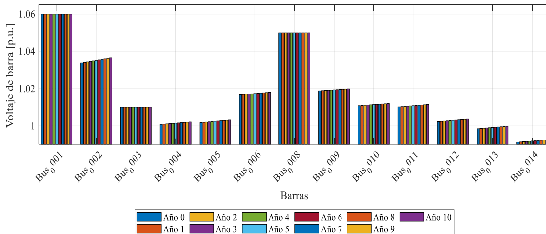
Figura 10. Voltajes de barra, sistema fotovoltaico de 60 MW.
